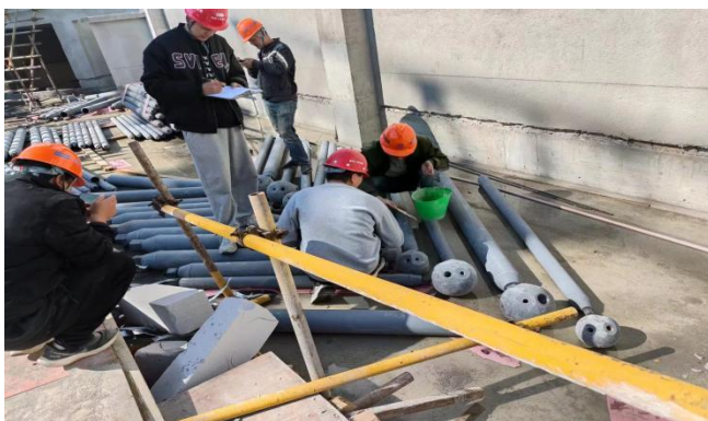
钢结构焊缝探伤检测及防火涂层厚度检测
